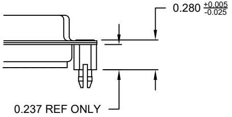
"90" // PCB SIDE **
